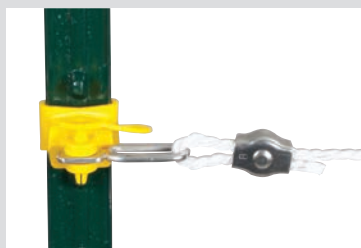
Anfangsbefestigung für Seil oder Litze mit Einhängelasche 1-fach
