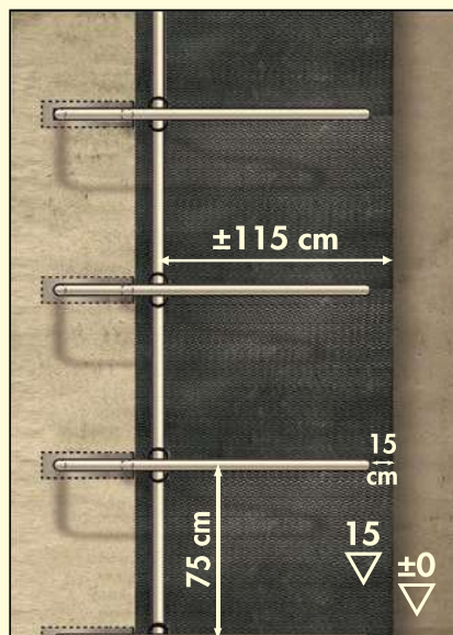
Maße Liegeboxenmontage Kälber
