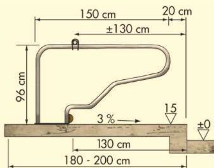
Hochbox
