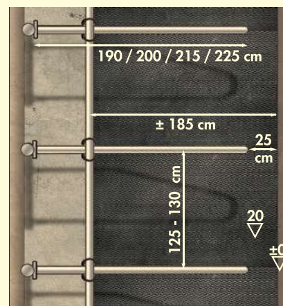
Variante 2: Montagemaße Liegeboxenbügel Universal Einzelreihe an Standpfosten für Großvieh, Beispiel Hochbox
