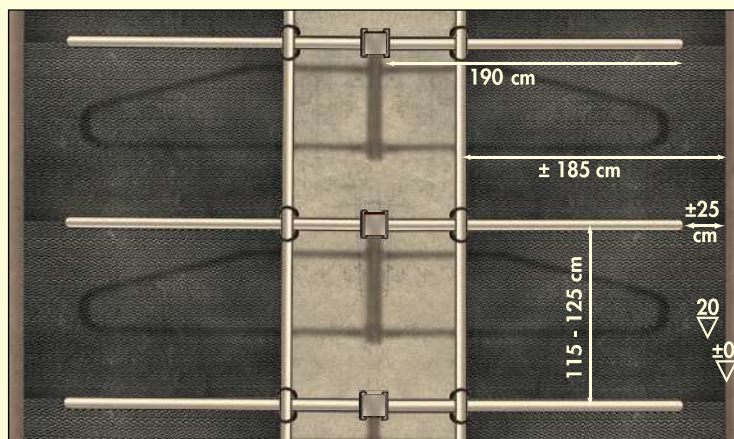
Variante 1: Montage Maße Doppelreihe flexibler Liegeboxenbügel an Standpfosten 60 x 60 mm für Großvieh, Beispiel Hochbox
