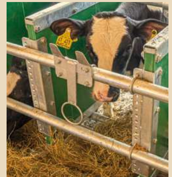
Höhenverstellbare Nuckeleimerhalter
