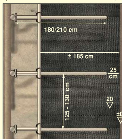
Maße Liegeboxenmontage Comfort für Großvieh
