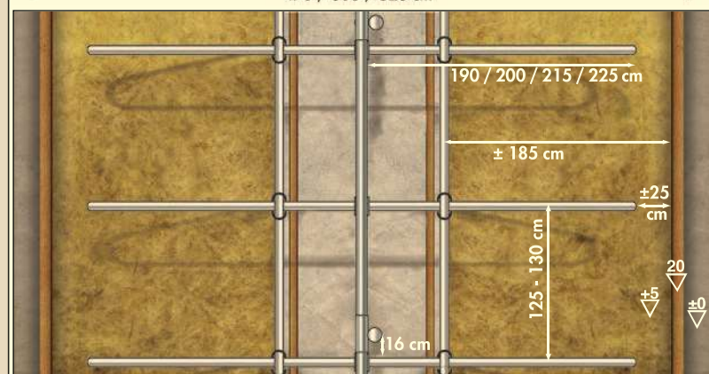
Variante 1: Montagemaße Liegeboxenbügel Universal Doppelreihe mit Trägergestell für Großvieh, Beispiel Tiefbox
