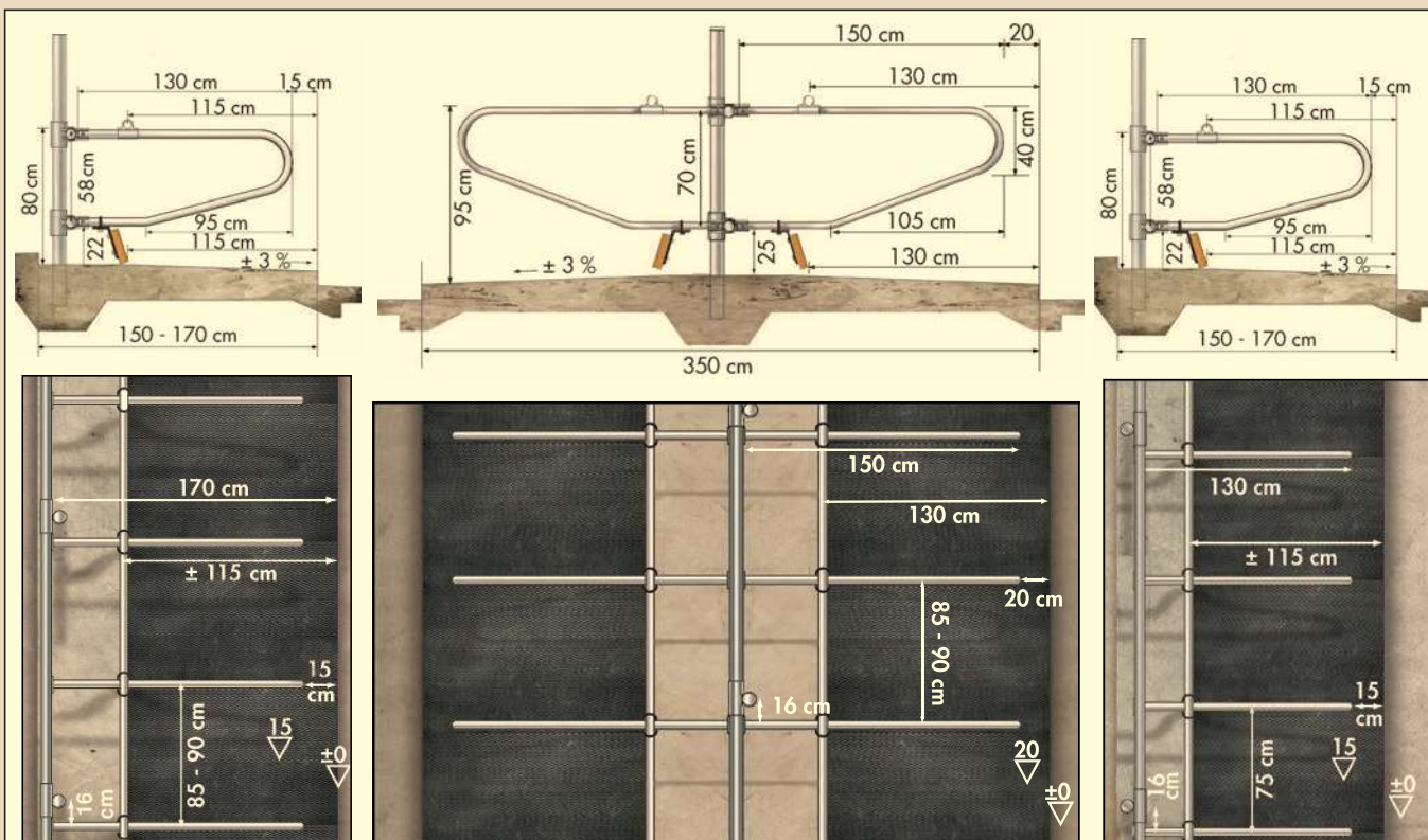
Variante 1: Montagemaße Liegeboxenbügel Universal Einzelreihe mit Trägergestell für Jungvieh
