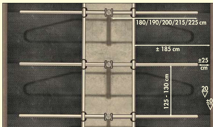
Variante 2: Montagemaße Liegeboxenbügel Universal Doppelreihe an Standpfosten für Großvieh, Beispiel Hochbox
