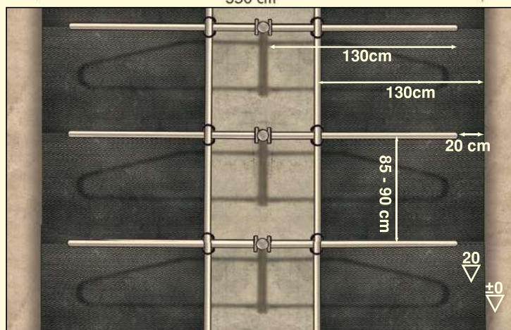
Variante 2: Montagemaße Liegeboxenbügel Universal Doppelreihe an Standpfosten für Jungvieh
