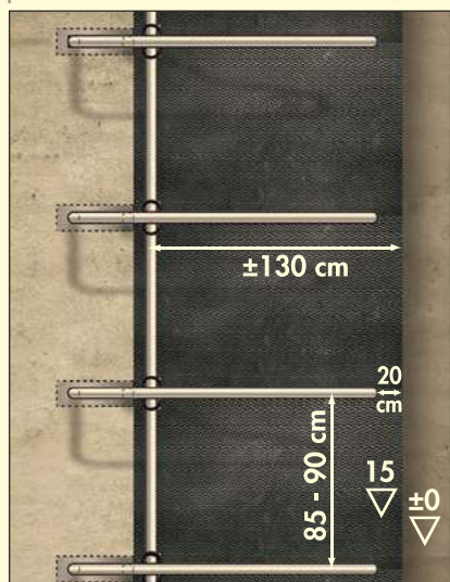
Maße Liegeboxenmontage Jungvieh
