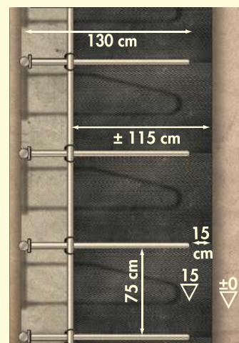
Variante 2: Montagemaße Liegeboxenbügel Universal Einzelreihe an Standpfosten für Kälber
