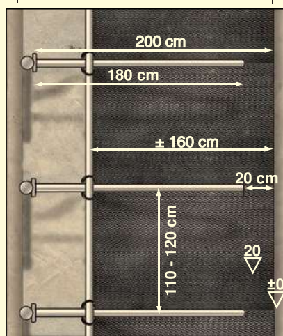
Maße Liegeboxenmontage Comfort für Färsen
