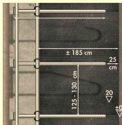
Variante 3: Montagemaße Liegeboxenbügel Universal Einzelreihe auf Montagebock für Großvieh, Beispiel Hochbox
