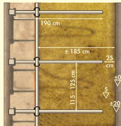
Variante 2: Montage Maße Einzelreihe flexibler Liegeboxenbügel, Beispiel Tiefbox
