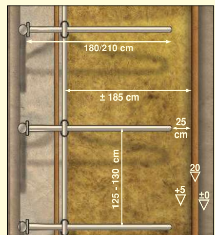
Maße Liegeboxenmontage Comfort für Großvieh
