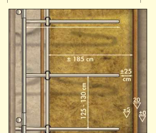
Variante 1: Montagemaße Liegeboxenbügel Universal Einzelreihe mit Trägergestell für Großvieh, Beispiel Tiefbox
