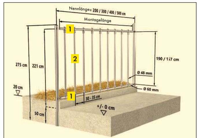
Modulares Pferdefressgitter mit Gitterstäben in Standard-Anordnung
