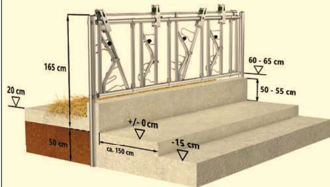
Montagehöhe Schwedenfressgitter
