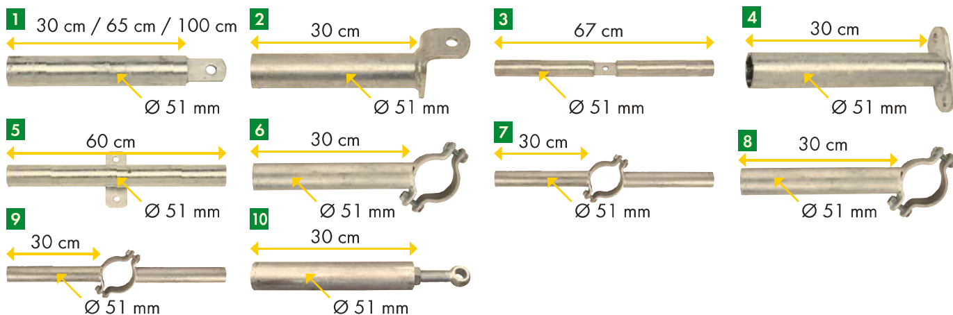
Untenauslass
