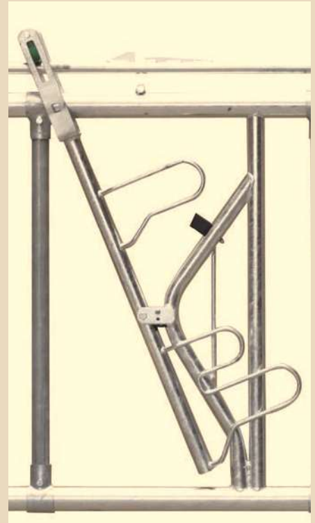
Position 3 Sicherheitsstellung „Notauslass“
