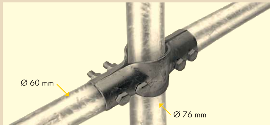
Aufbaubeispiel Ref. 341275
