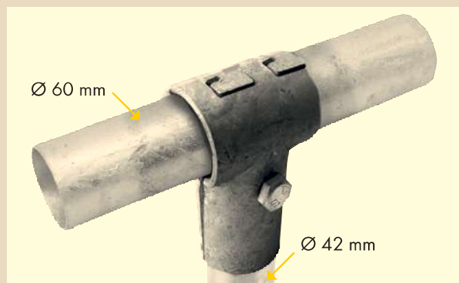
Aufbaubeispiel Ref. 341209
