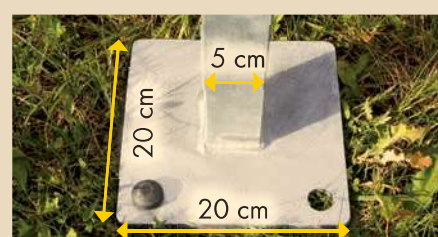
Standfüße ermöglichen eine sichere Verankerung mittels Erdnägeln
