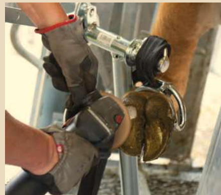
2 Klauenpflege mit rückschlagfreien Winden
