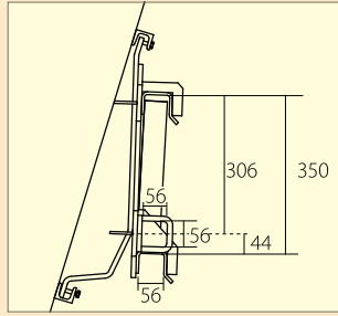
6. Schäffer-Hoflader mechanische Verriegelung, obere Einhänghöhe: 966 mm
